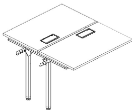
PLATAFORMA ACOPLAR DUPLA SMART PROF. 1400 MM
