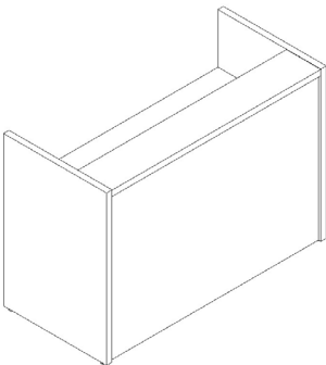
BALCÃO ATENDIMENTO ALTO
